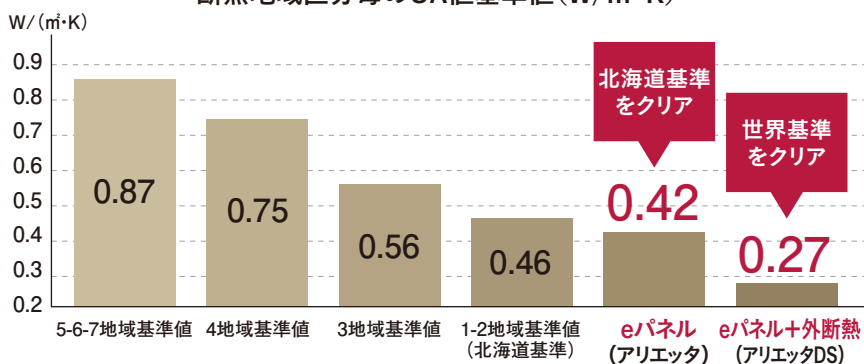
断熱地域区分毎のUA値基準値(W/m 2 ・K)
